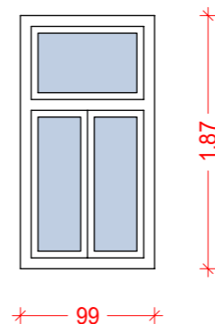
O1 Okno - dim. 99 x 187 cm 10 kosov Pritličje 3x ( po opisu iz POPISOV DEL ) Nadstropje 7x ( po opisu iz POPISOV DEL )
