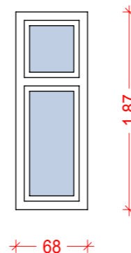
O2 Okno - dim. 68 x 187 cm 3 kosi Pritličje 2x ( po opisu iz POPISOV DEL ) Nadstropje 1x ( po opisu iz POPISOV DEL )
